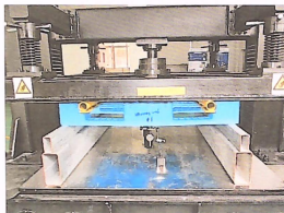
抗弯强度图片 (长方向)
