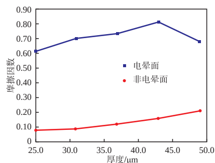
图1 薄膜厚度对CPP热封膜摩擦因数的影响
