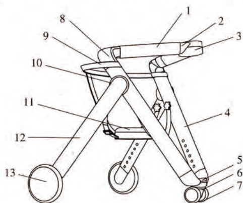
1 EVA 包裹料; 2 铝制扶手; 3 顶部转轴; 4 前支撑管; 5 底部转轴; 6 前轮轴; 7 前轮; 8 ABS 连接件; 9 后背绑带; 10 中间转轴; 11 坐垫; 12 后支撑管; 13 后轮
